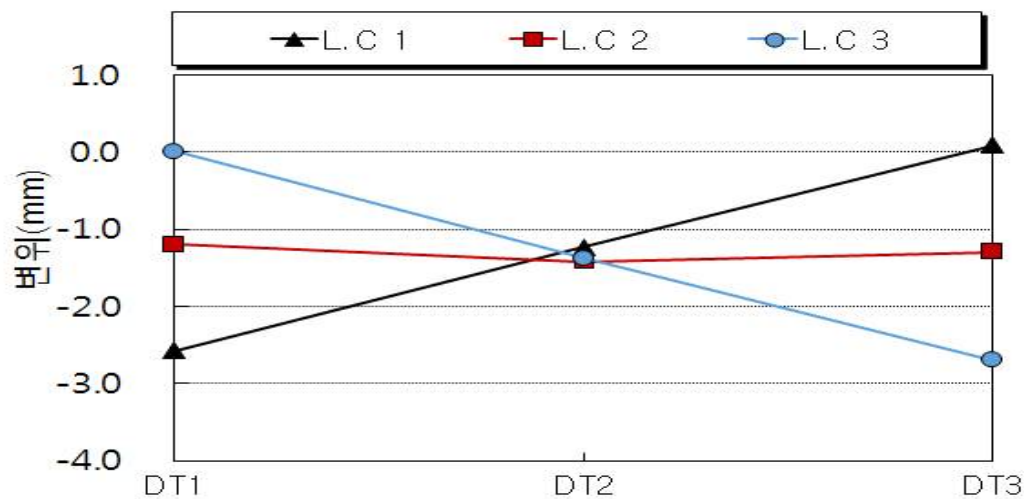
처짐 횡분배 현황
