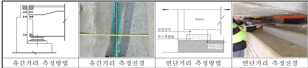
【그림 2.6.10】 부재별 기능상태 측정방법 및 전경
