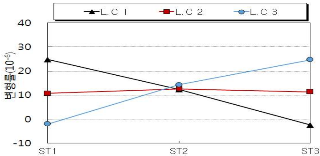
변형률 횡분배 현황
