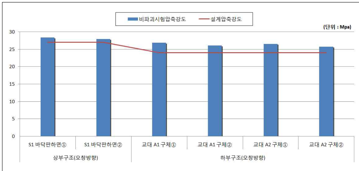
【그림 2.6.11】 콘크리트 강도시험 결과 그래프
